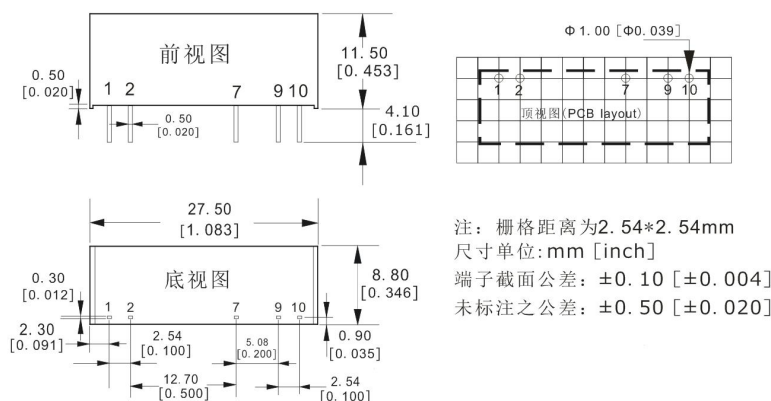
封装尺寸图
